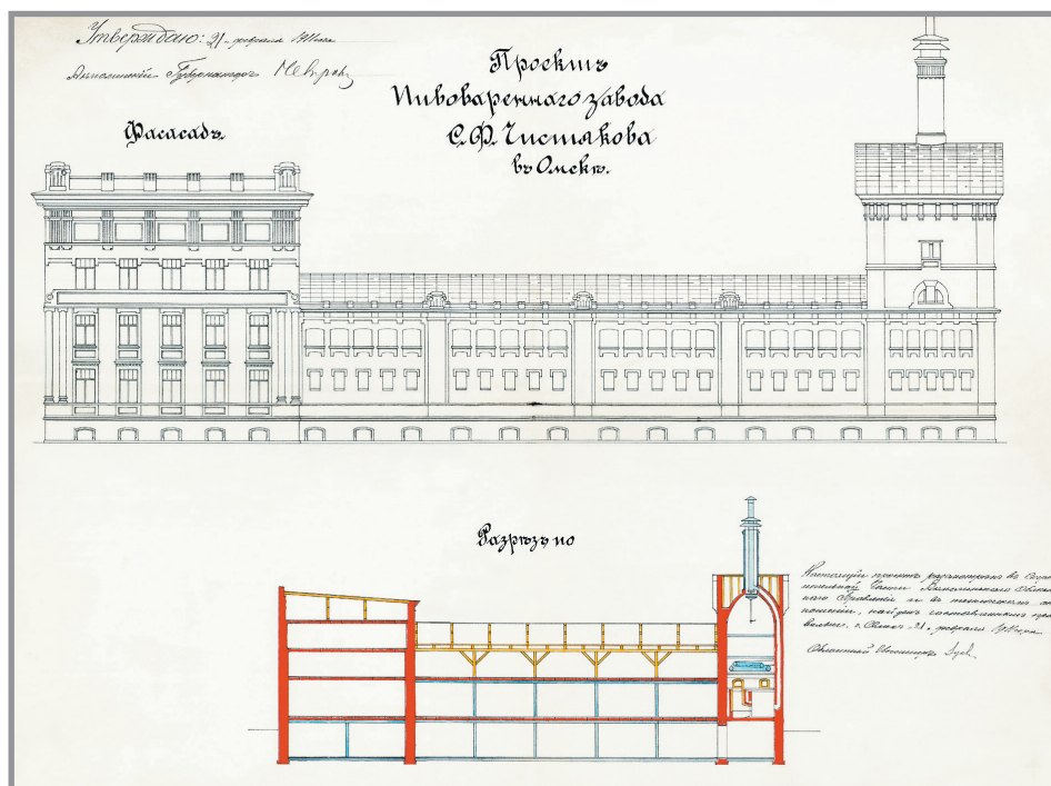
Проект пивоваренного завода купца С. Ф. Чистякова, основного конкурента купца А. Ф. Поклевского-Козелла в Омске. Из фондов ГИАОО
