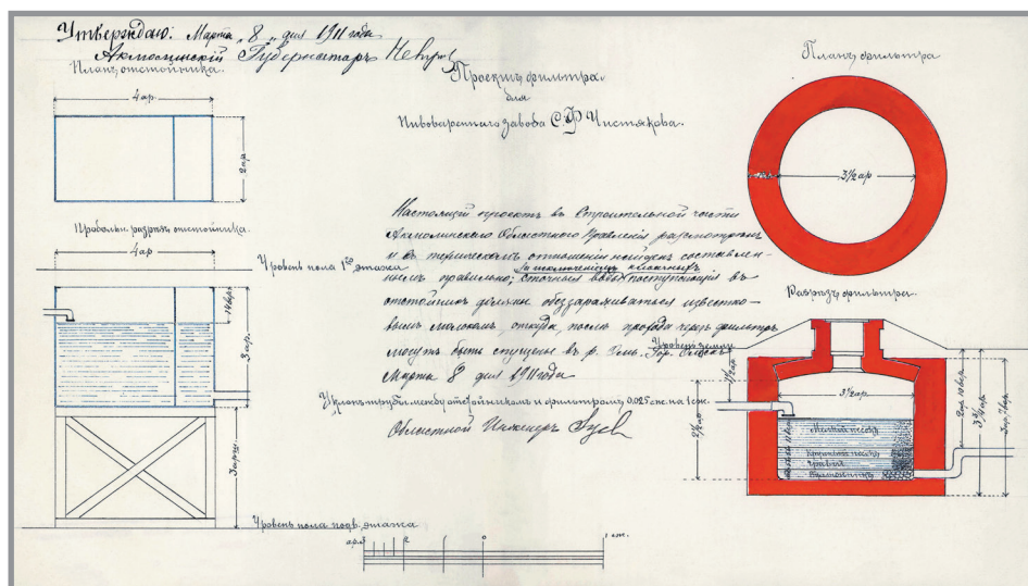
Проект фильтра для пивоваренного завода купца С. Ф. Чистякова. Из фондов ГИАОО
